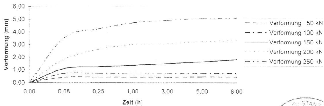
Distanzplatten 70 x 70 , d = 15 mm
