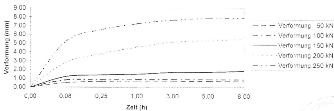
Distanzplatten 70 x 70 , d = 20 mm
